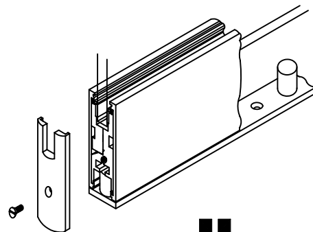
Modulschiene für Seitenteil
